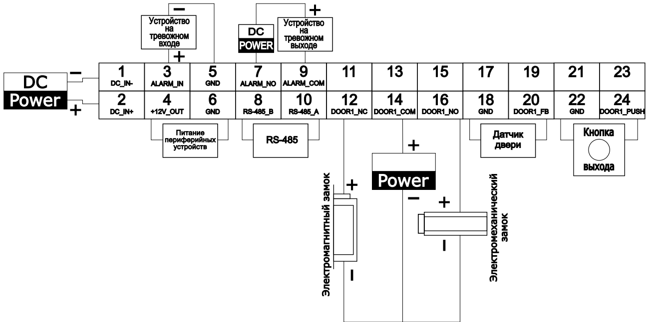
Рисунок 3.3 – Схема подключения. Замок 1
