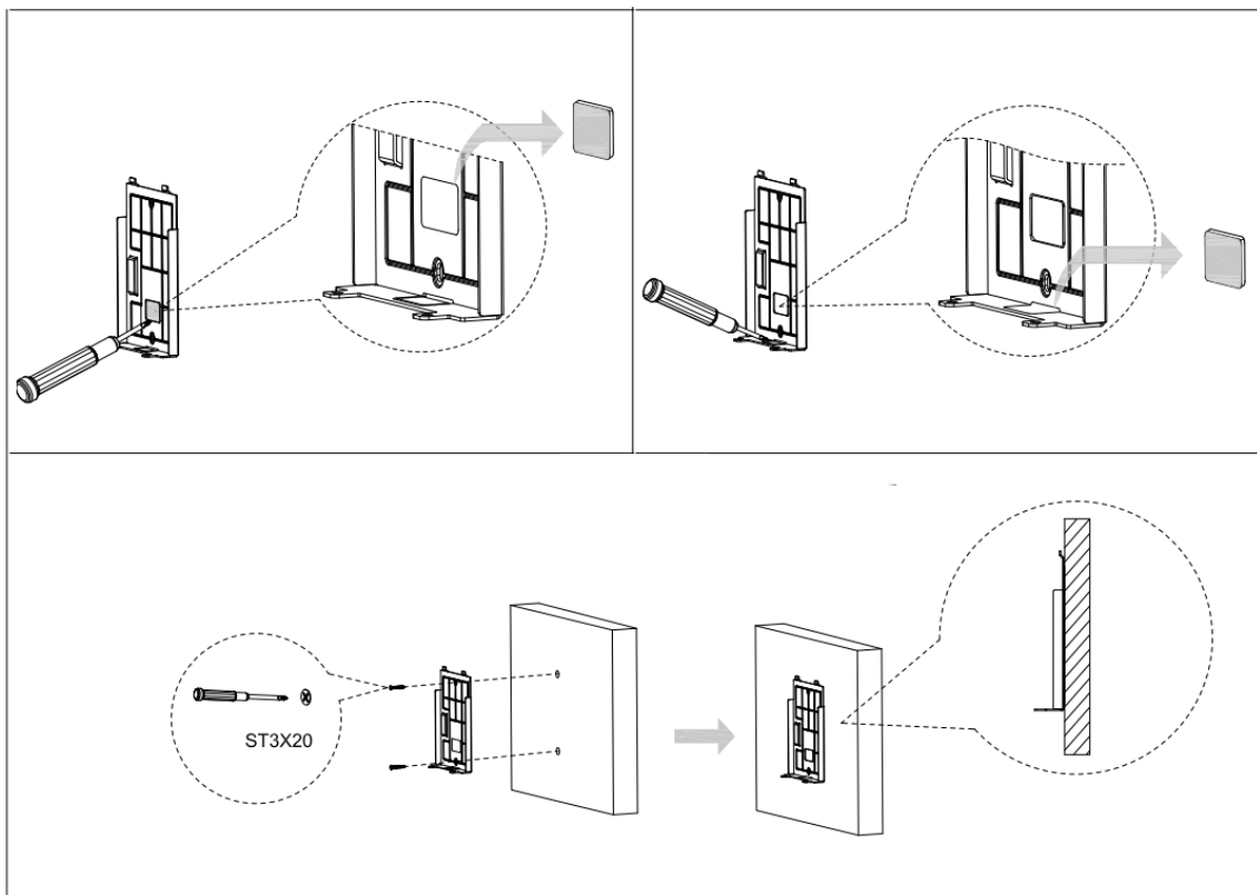
Рисунок 4.6 – Схема установки
