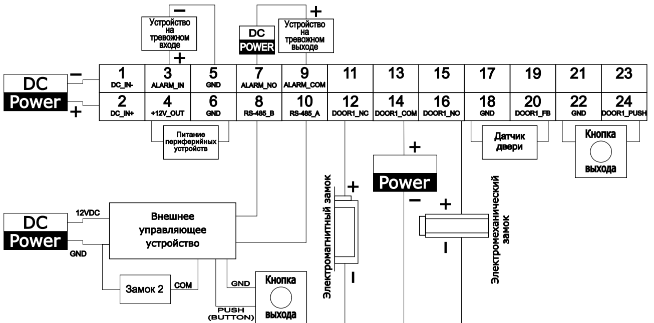
Рисунок 3.4 – Схема подключения. Замок 2
