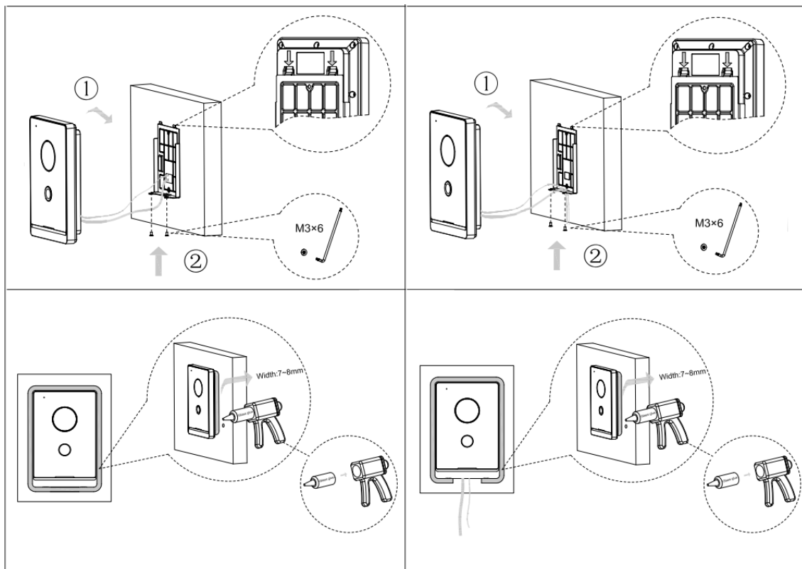
Рисунок 4.8 – Схема установки
