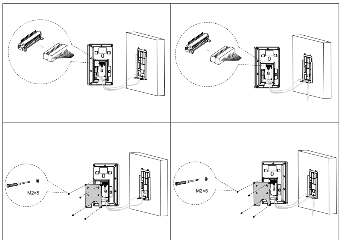
Рисунок 4.7 – Схема установки
