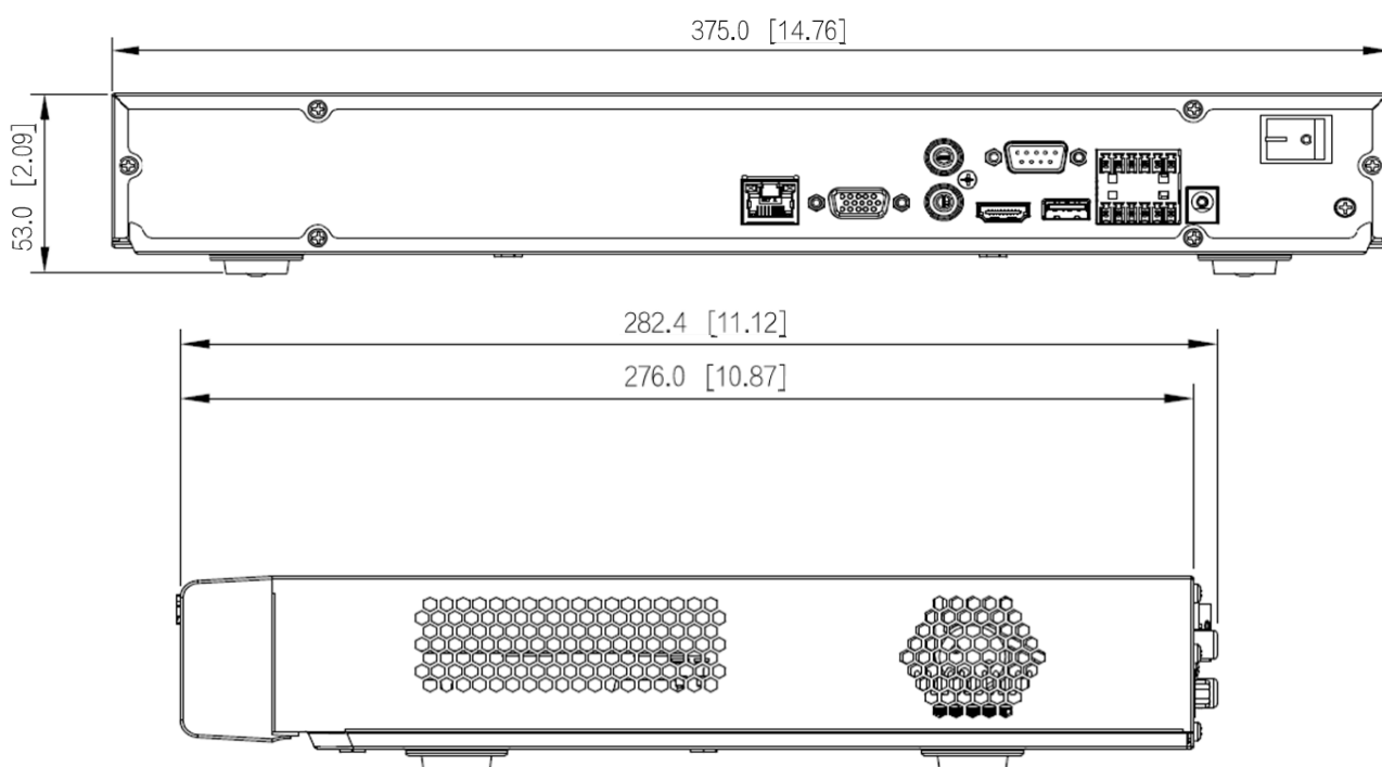
Рисунок 3.9 – Габаритные размеры видеорегистратора
