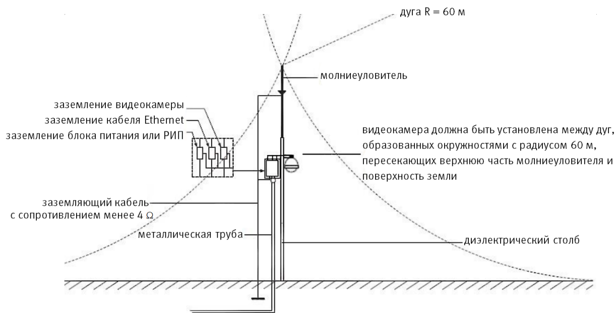
Рисунок 8.4 – Установка молниеотвода
