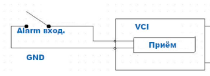
Рисунок 6.6 – Схема подключения тревожного входа
