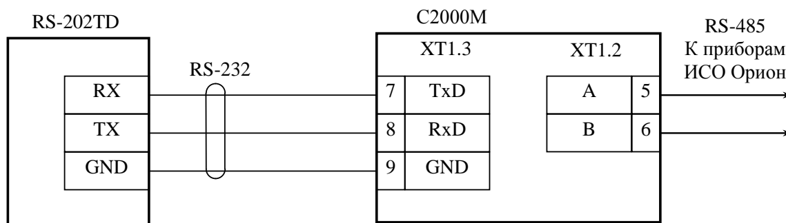
RS-202TD – радиопередатчик «Риф Стринг RS-202TD-RR»; С2000М - пульт контроля и управления «С2000М».
