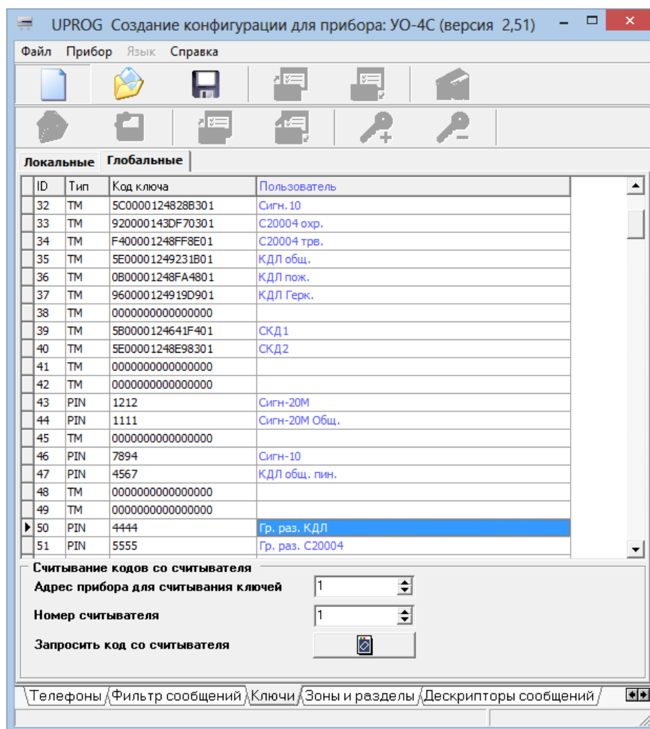
Рисунок 16. Глобальные ключи, мастер режим
