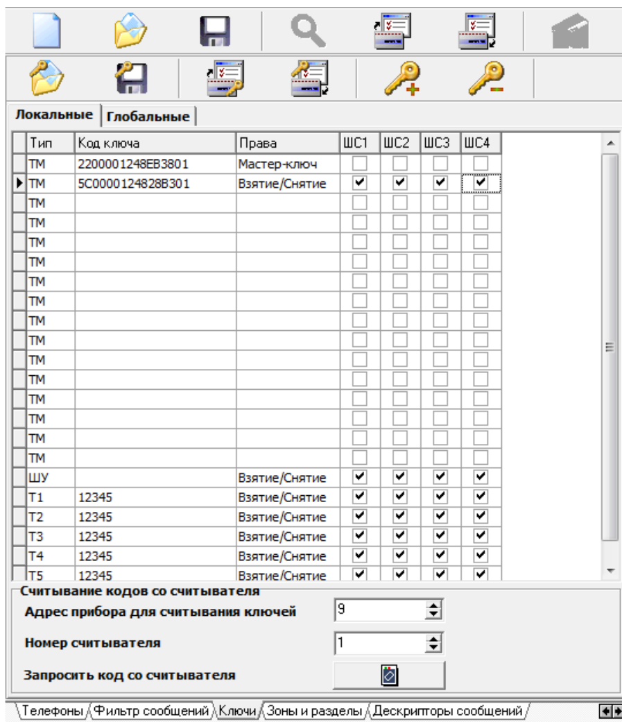
Рисунок 15. Локальные ключи
