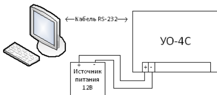
Рисунок 7. Подключение «УО-4С» к ПК через кабель сопряжения
