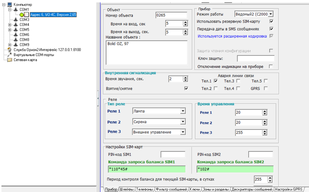
Рисунок 10. Uprog «УО-4С»
