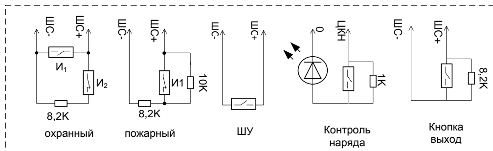
Рисунок 4. Подключение ШС, ШУ
