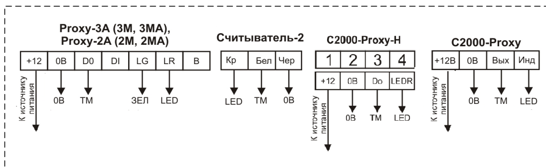
Рисунок 5. Подключение считывателей
